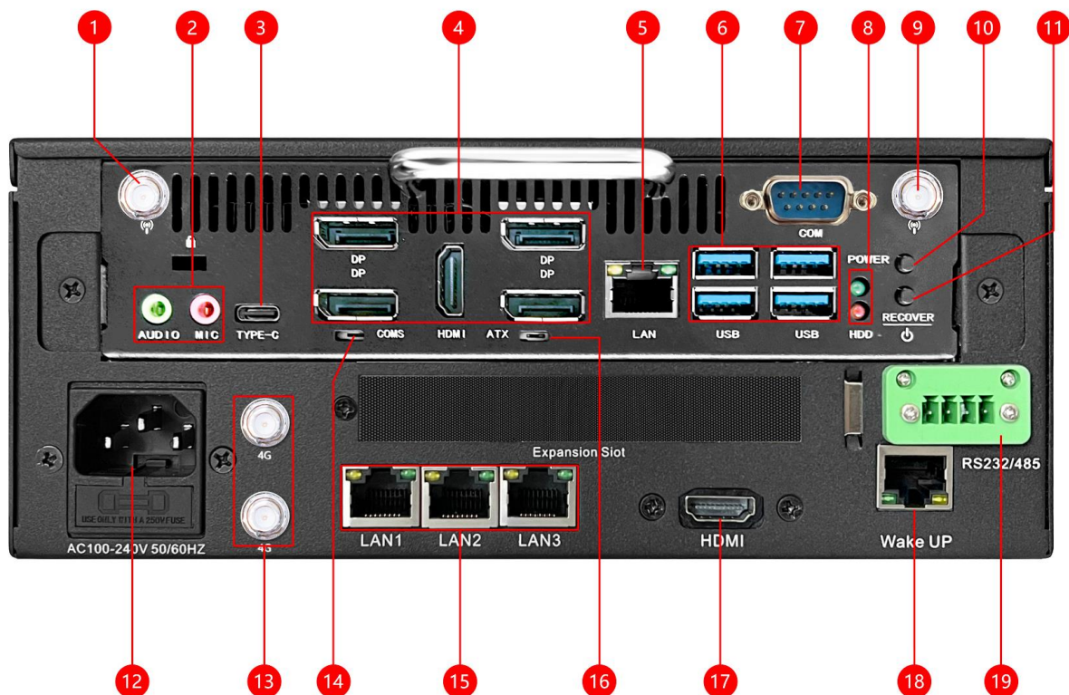
后面板
